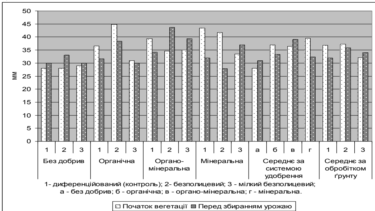
Рис. 1 Запаси доступної води в (0–30 см) шарі ґрунту, мм
